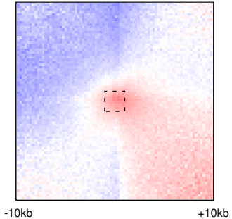
ED (n=179333)
