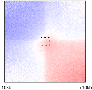
Embryo (n=179333)
