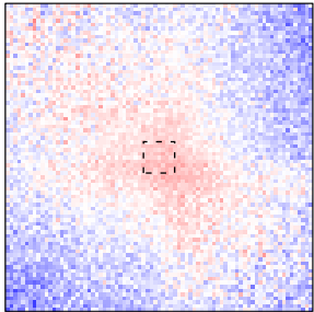
Embryo (n=4274)
