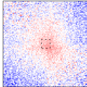
WD (n=4274)
