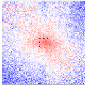
ED (n=4274)
