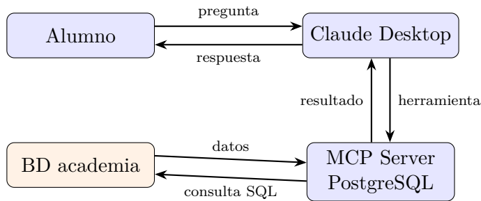
Figura 13.2: Flujo de una consulta con MCP
