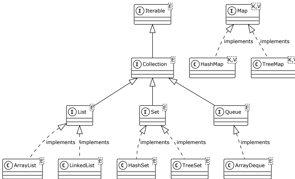
Figura 14.1: Jerarquía del Java Collections Framework
