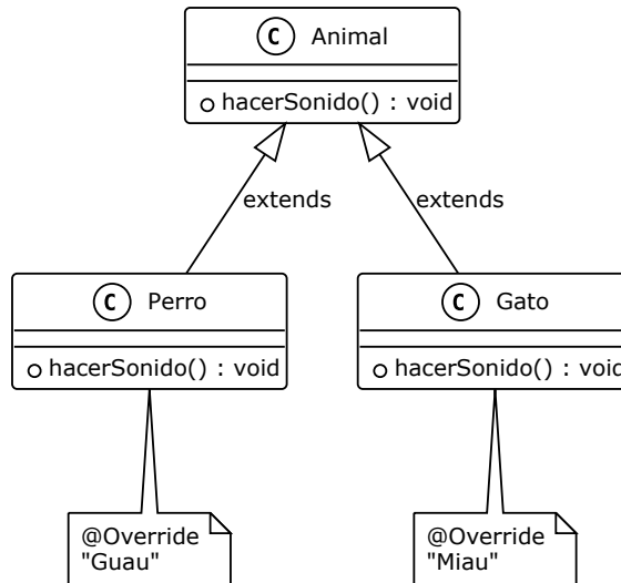
Figura 15.2: Polimorfismo: Perro y Gato sobrescriben hacerSonido()
