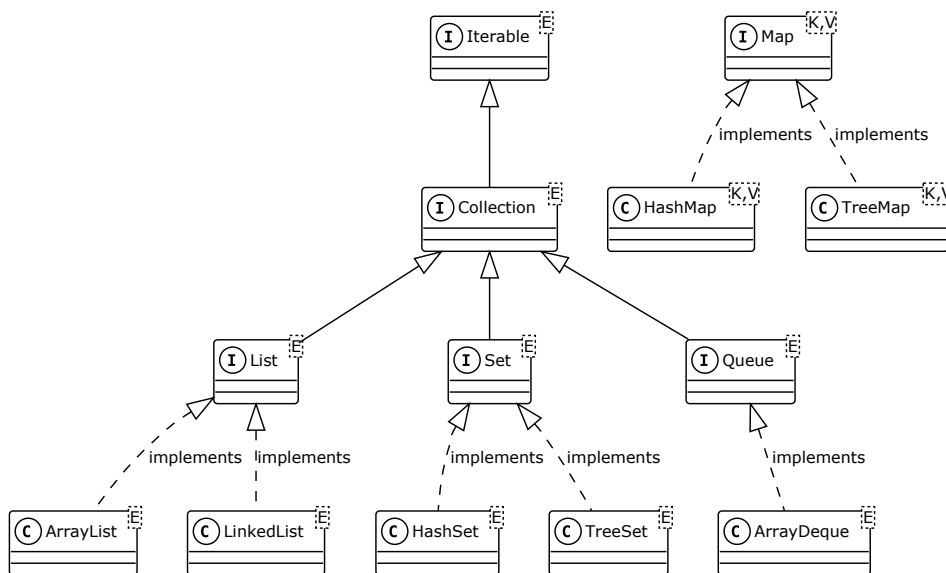
Figura 13.1: Jerarquía del Java Collections Framework
