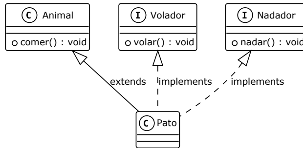
Figura 15.3: Herencia e implementación de interfaces: Pato extiende Animal e implementa Volador y Nadador
