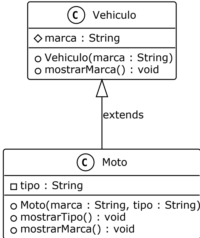
Figura 9.1: Diagrama de clases: herencia de Vehiculo a Moto
