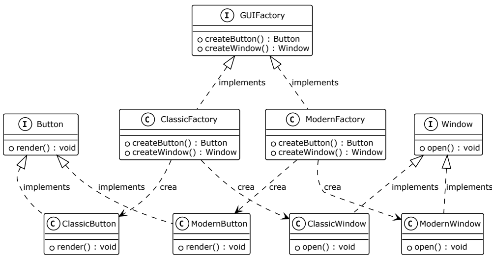
Figura 21.1: Diagrama UML del patrón Abstract Factory
