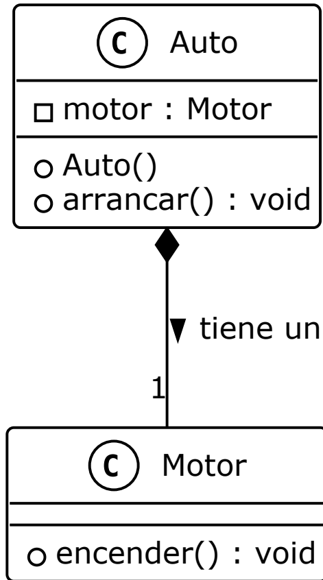
Figura 15.1: Diagrama de composición: Auto contiene un Motor
