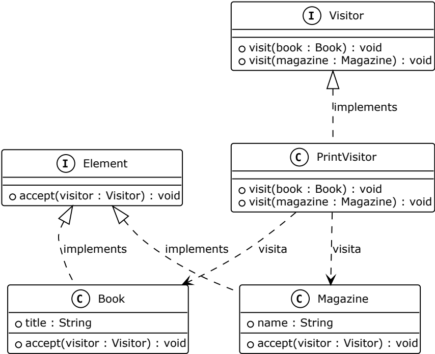
Figura 21.3: Diagrama UML del patrón Visitor
