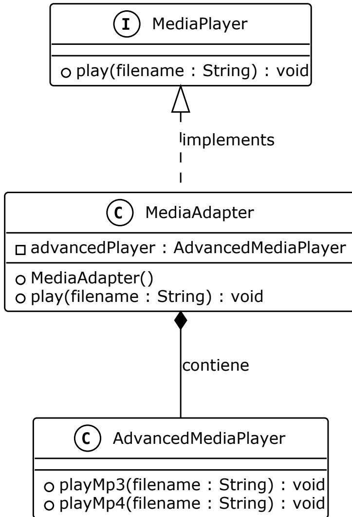
Figura 21.2: Diagrama UML del patrón Adapter
