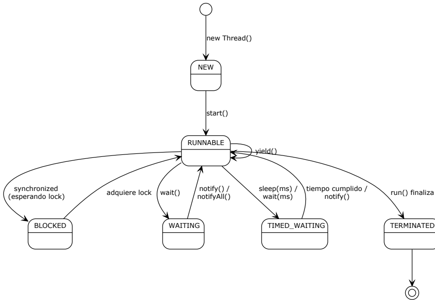
Figura 22.1: Ciclo de vida de un hilo en Java
