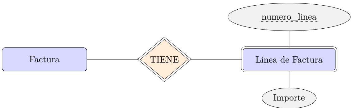
Figura 5.5: Transformación de entidad débil
