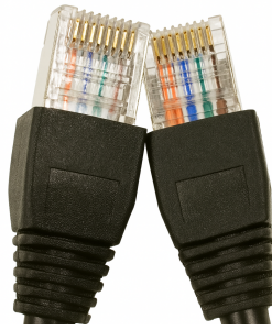
Figura 4.13: Ejemplo de un cable que usa el estándar T568B
