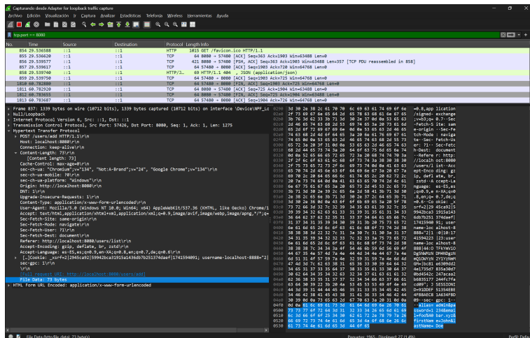
Figura 8.1: Wireshark, una herramienta popular para la captura y análisis de tráfico de red.
