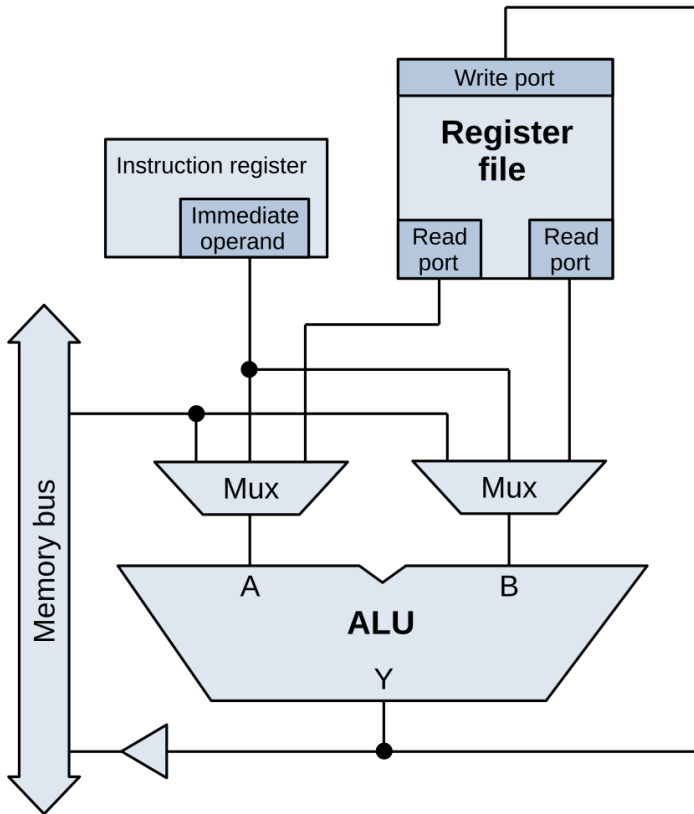
Figura 4.2: Diagrama de un procesador
