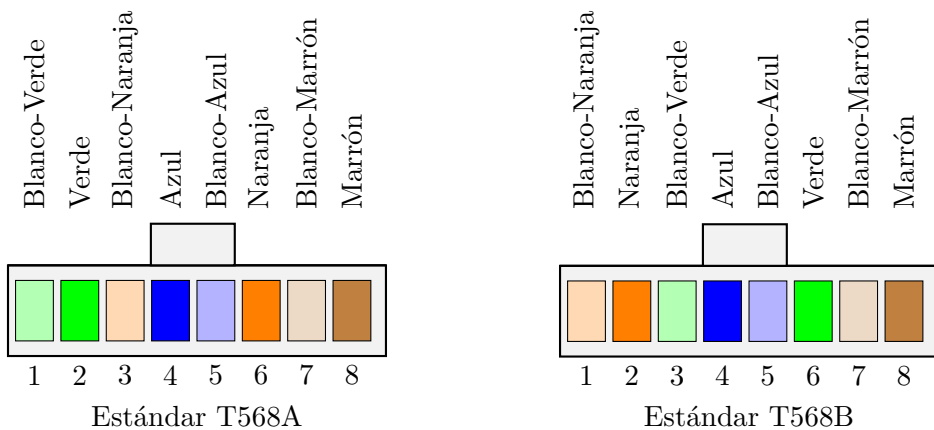
Figura 4.12: Distribución de hilos en un conector RJ45
