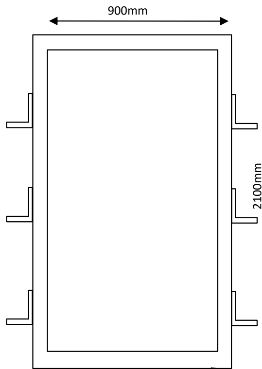
DOOR CHOWKAT
