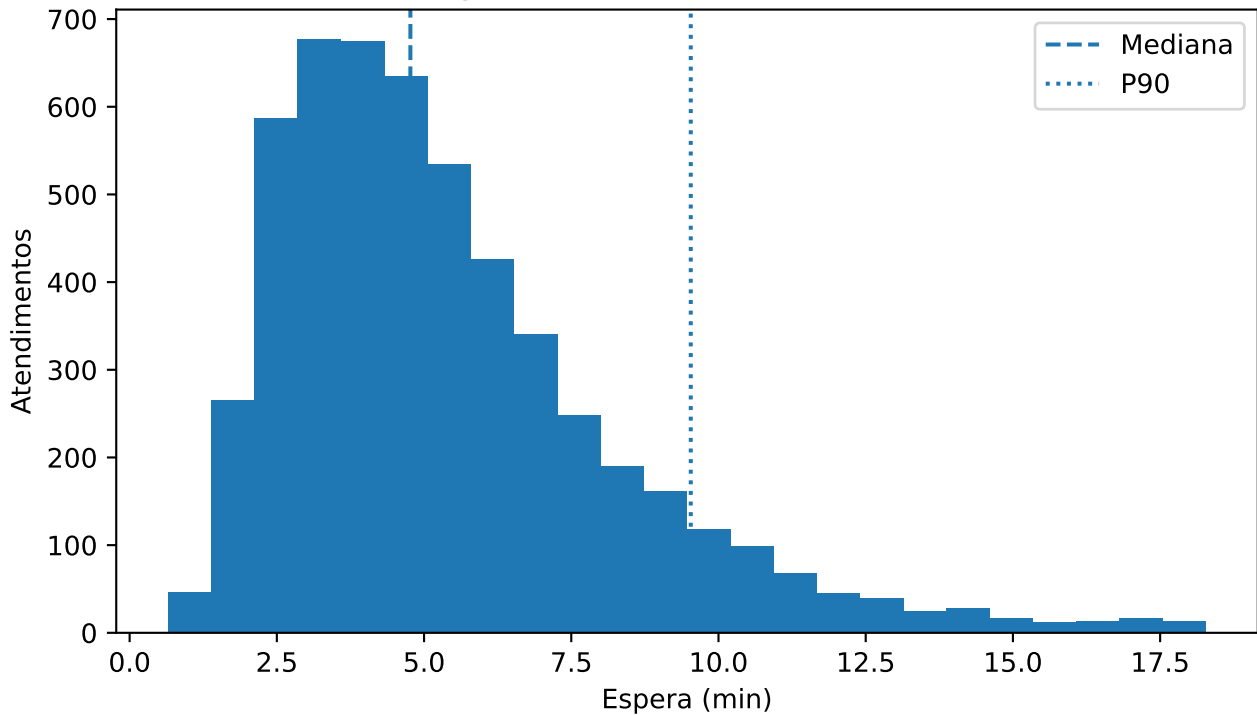
Histograma: forma, assimetria e cauda
