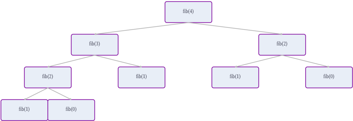
圖解三：費氏數列 — 遞迴為何慢（以 fib(4) 展開）
