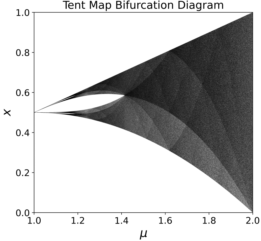
Figura 4: Estados de la familia T_\mu después de 1000 iteraciones.
