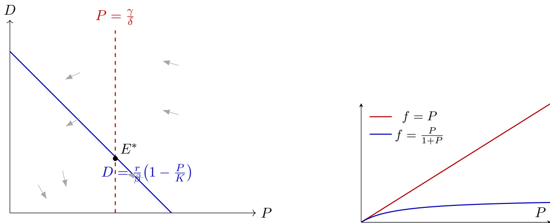
Figura 32: Plano de fases presa-depredador (versión generalizada con capacidad de carga) y respuestas funcionales típicas: lineal f = P (Lotka-Volterra clásico) y saturada f = P/(1 + P) (Holling tipo II).
