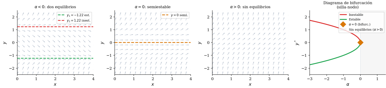
Figura 15: Campos de pendientes y diagrama de bifurcación silla-nodo de y' = y^2 + \alpha .
