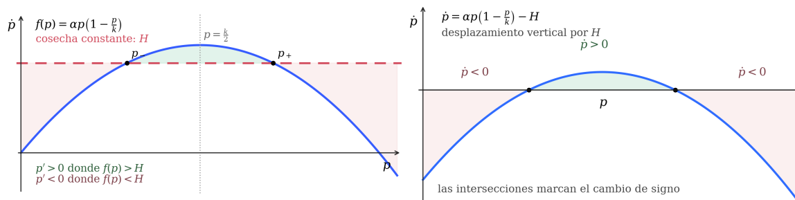
Figura 33: Izquierda: curva de crecimiento logístico f(p) y recta de cosecha H . Derecha: función neta p' = f(p) - H con sus ceros y signos. Los ceros son los equilibrios y su estabilidad se lee del signo de la derivada.
