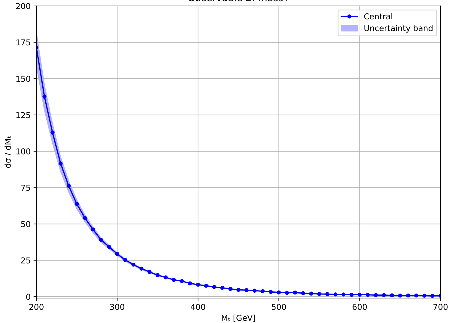
Observable 2: \text{massT}
