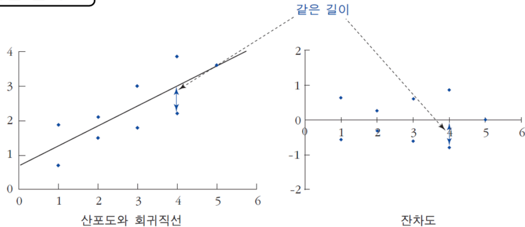
일반적인 잔차도
