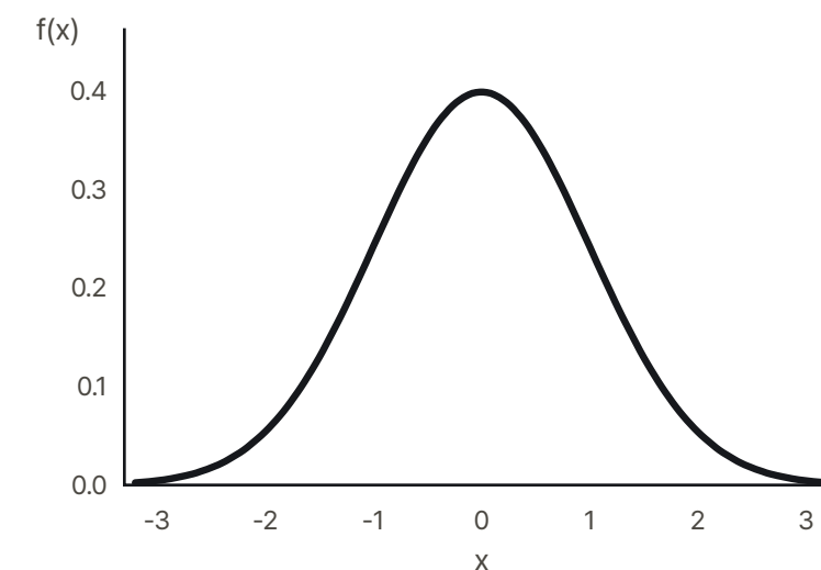
연속변수의 히스토그램
