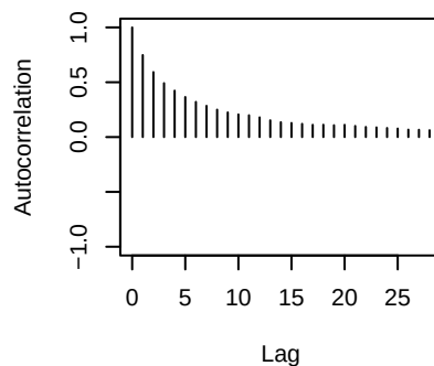
lambda[9]
