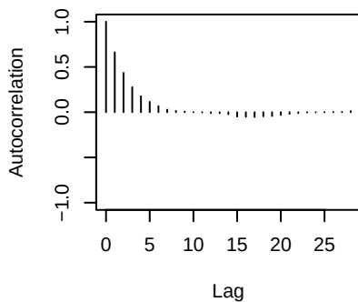
lambda[5]
