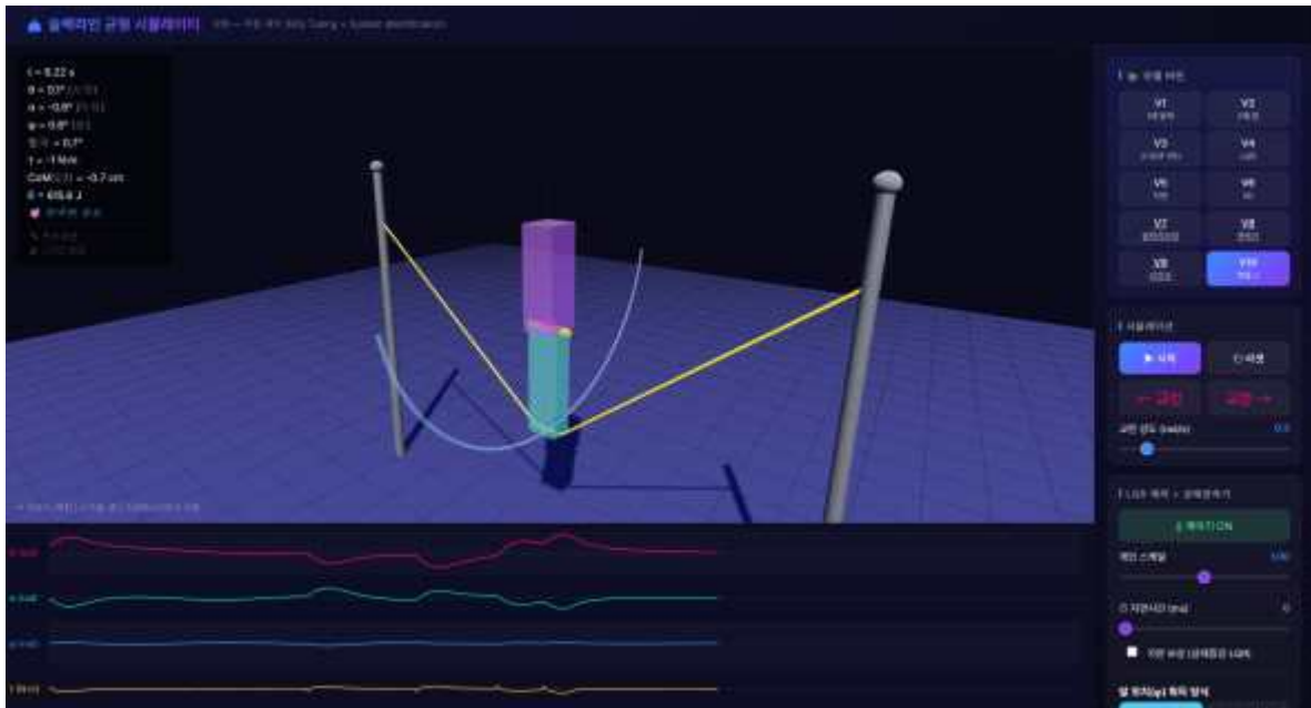
그림 33 LQR제어 시뮬레이션
