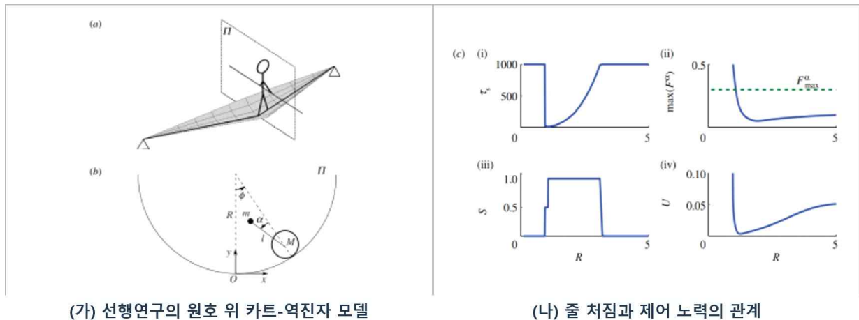
그림 2. Paoletti와 Mahadevan의 선행연구: 원호 위 카트-단일 역진자 모델과 줄 처짐에 따른 제어입력의 변화.
