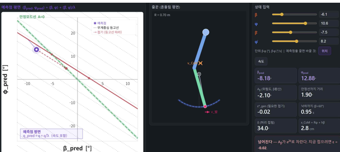
그림 29 기다리는 상태
