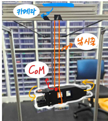
그림 43 비틀림 진자로 관성모 먼트 실측
