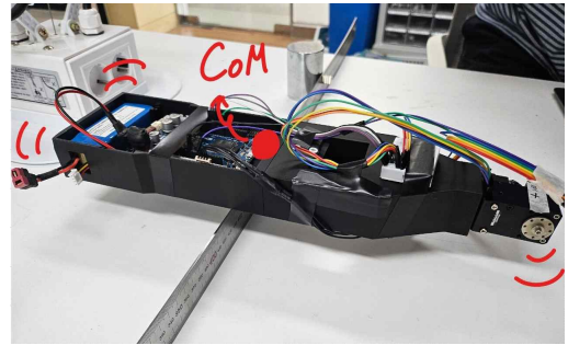
그림 44 나이프 엣지 방법으로 무게중심 위치 측정
