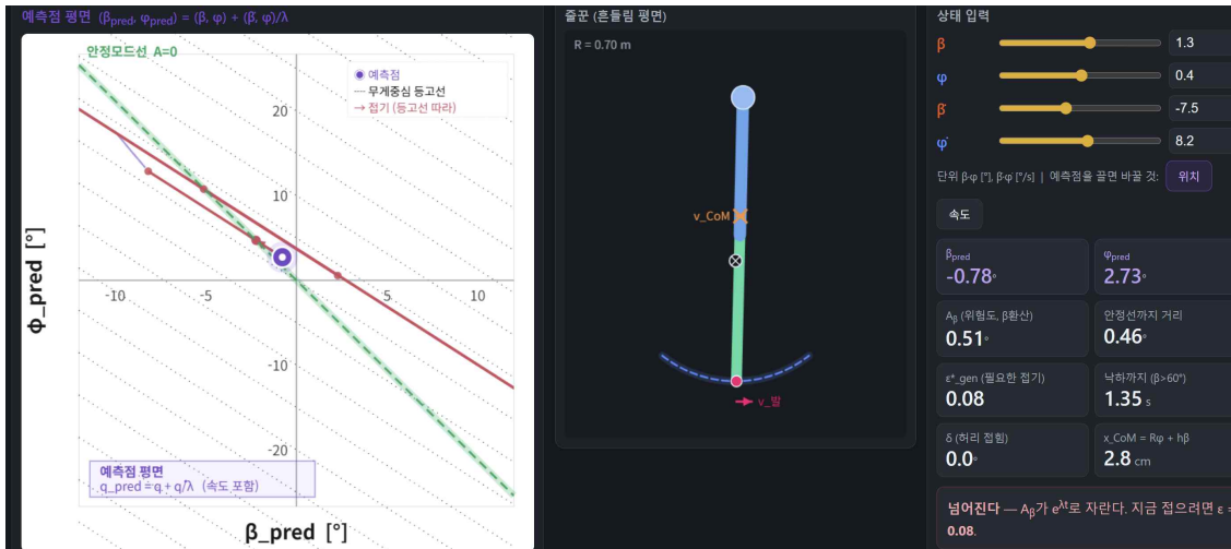
그림 30 몸을 편 후 안정 모드션 위에 있는 상태 이제 상태공간을 하나로 나타내 주면 다음과 같은 그림이 나오게 된다.
