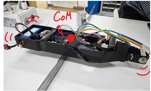
그림 44 나이프 엣지 방법으로 무게중심 위치 측정
