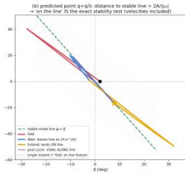
그림 31 FWE완전 사이클을 \beta_{pred}, \phi_{pred} 위에 나타낸 상태
