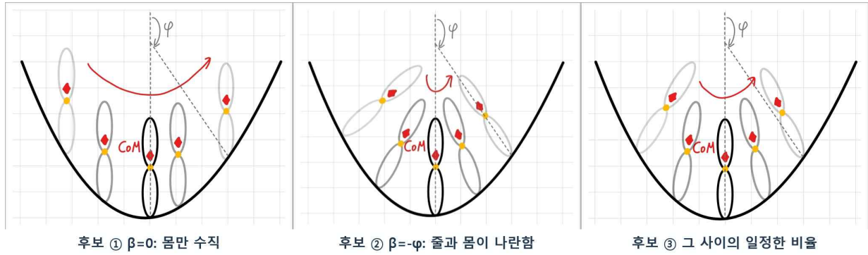
그림 6. 입력 없이 떨어지지 않는 운동을 찾기 위한 세 후보: \beta=0 , \beta=-\phi , 그리고 그 사이의 일정한 비율.
