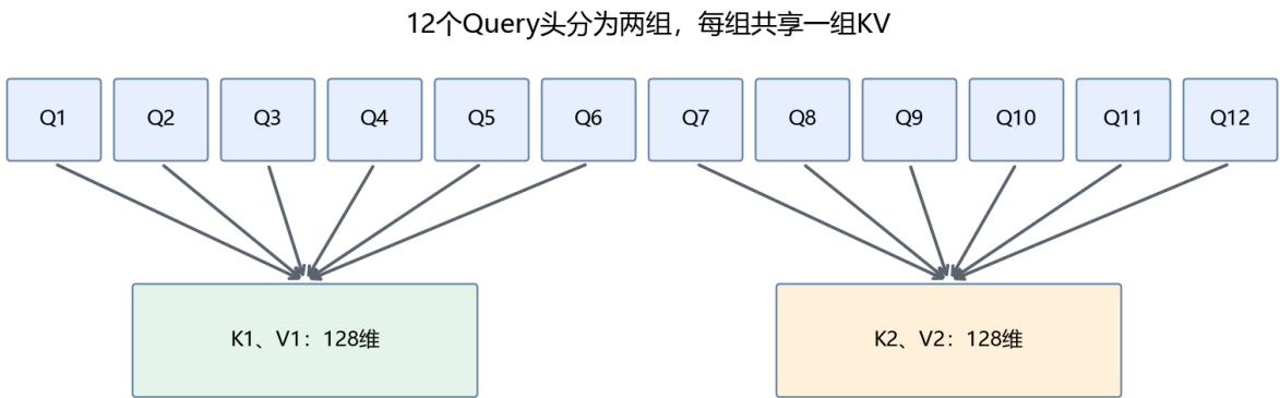
KV缓存保存2个头的历史Key和Value，不保存12份重复数据
