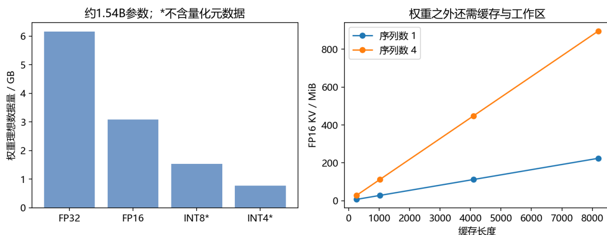
推理内存的主要组成
