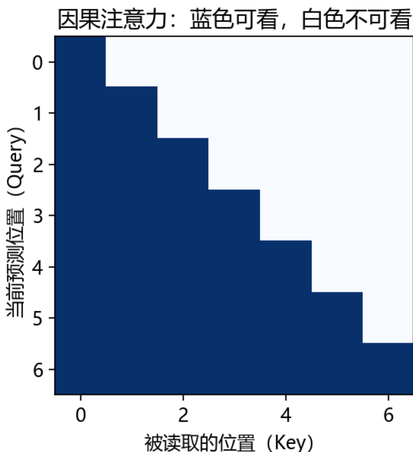
因果掩码
