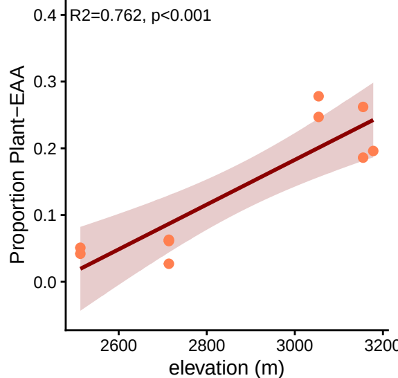
Copepoda
