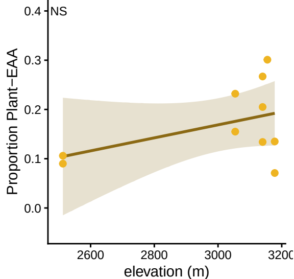
Cladocera
