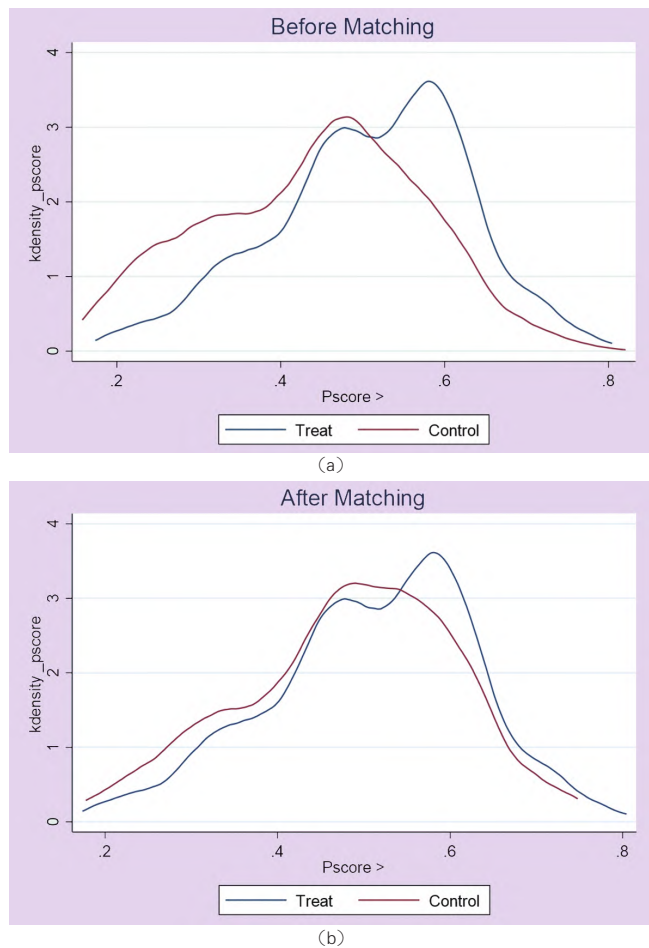
图1 匹配前后核密度函数曲线
