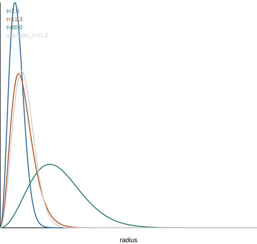
F. Radial van Hove vs Gaussian
