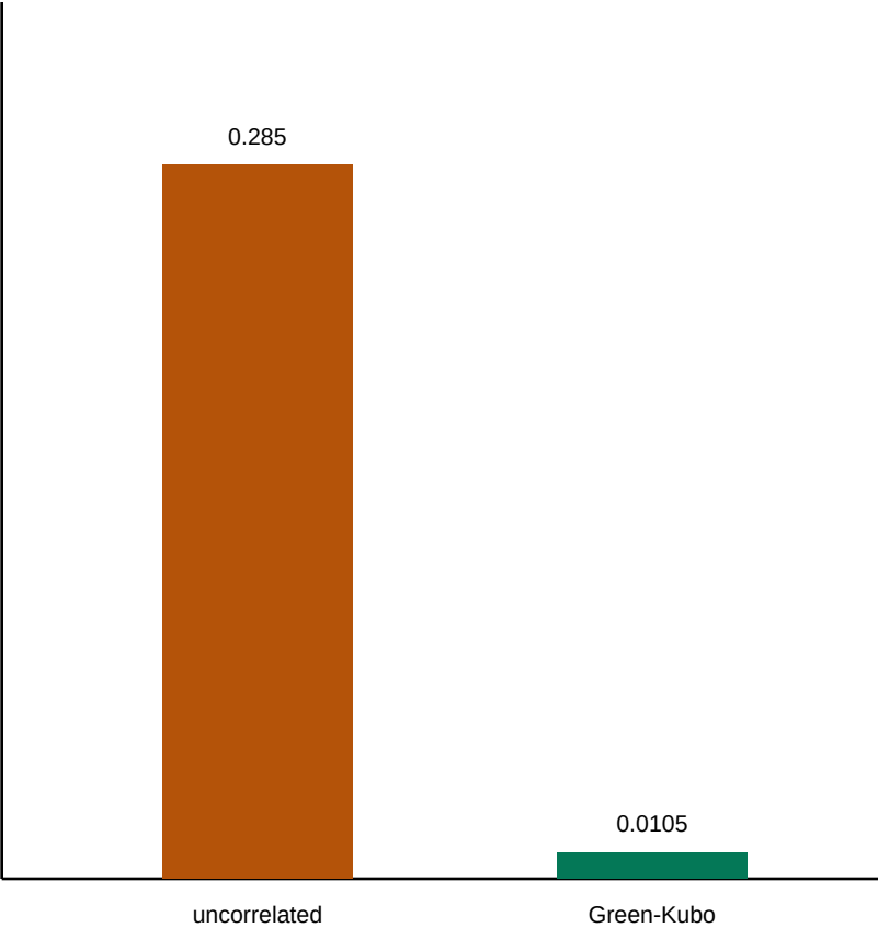
A. T=0.45 diffusion relative error
