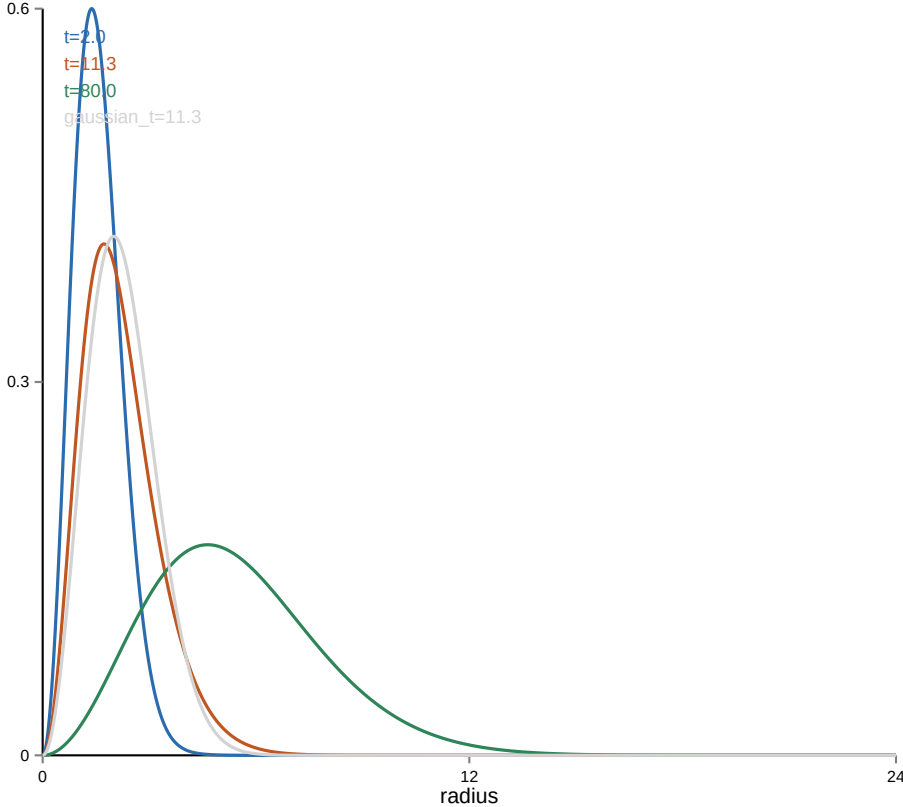
F. Radial van Hove vs Gaussian
