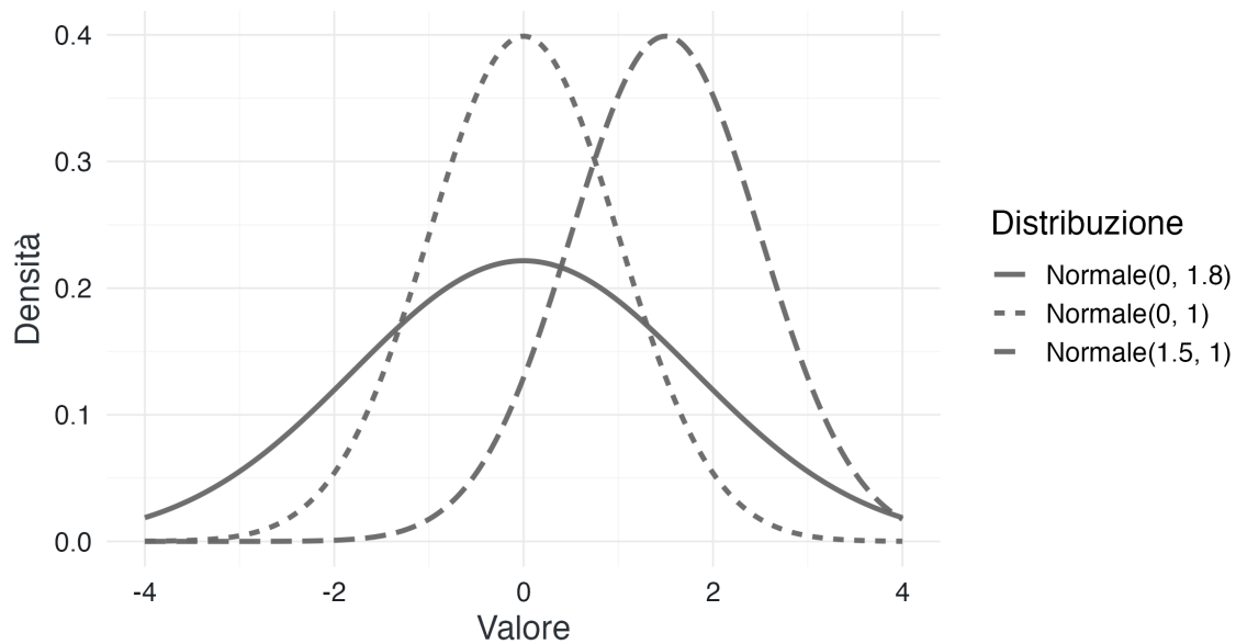
Figura 10.1.: Effetto dei parametri di posizione e scala nella famiglia normale. La media sposta il centro della distribuzione; la deviazione standard ne modifica la dispersione.
