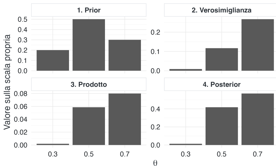
Figura 15.1.: Aggiornamento bayesiano su tre valori possibili. Il prodotto punto per punto ripesa la prior; la normalizzazione produce la posterior. Le scale verticali sono separate perché le quattro quantità hanno ruoli differenti.
