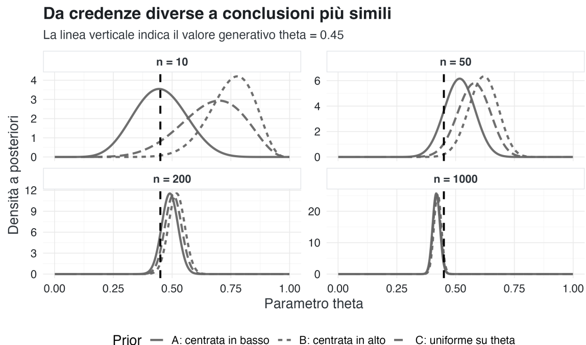
Figura 13.5.: Distribuzioni posteriori ottenute con prior diverse ma con gli stessi dati cumulativi, al crescere della dimensione campionaria.
