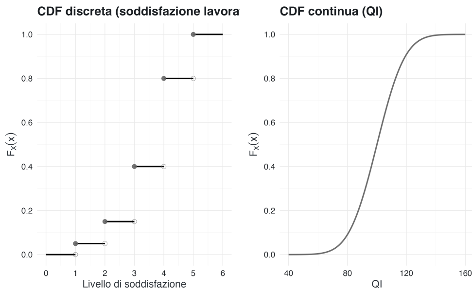
Figura 7.3.: CDF di una variabile discreta (sinistra, a gradini) e di una variabile continua normale (destra, curva liscia). Nella CDF discreta, l'ampiezza di ogni salto corrisponde alla massa nel punto.
