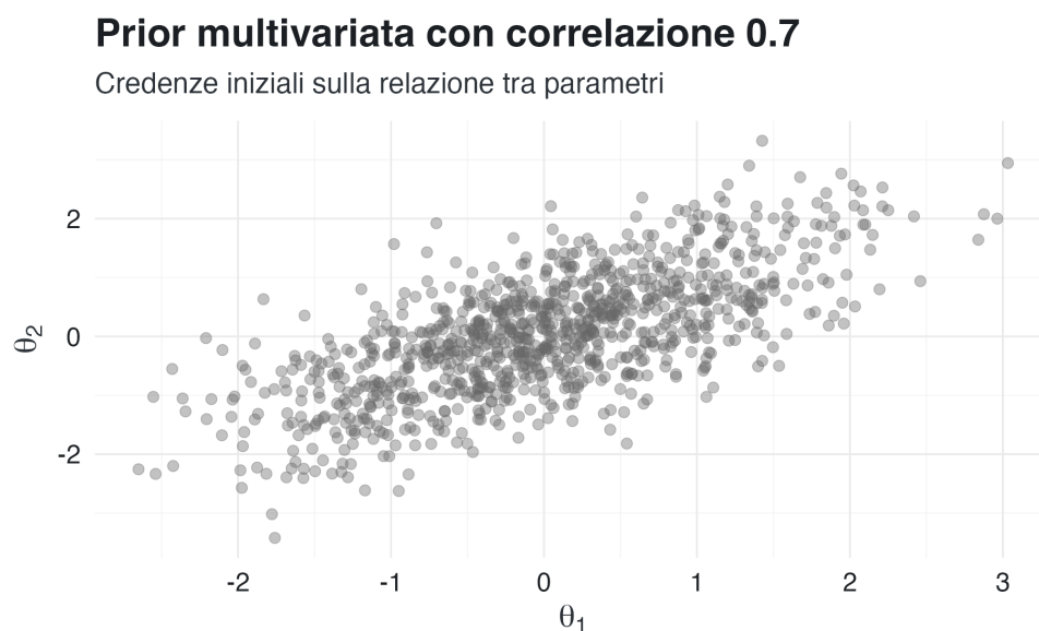
Figura 9.3.: Campioni da una distribuzione a priori bivariata con correlazione positiva tra i due parametri.
