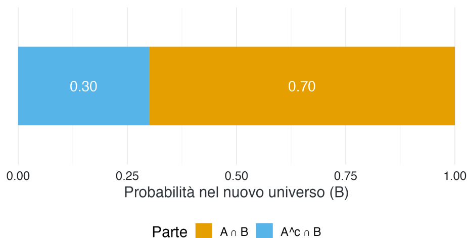
Figura 4.1.: Il condizionamento restringe lo spazio a B e rinormalizza le probabilità al suo interno.
