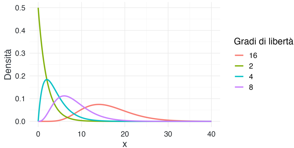
Figura 12.6.: Distribuzioni chi-quadrato con diversi gradi di libertà.
