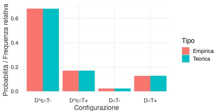
Figura 2.3: Confronto tra probabilità teoriche e frequenze relative ottenute dalla simulazione.
