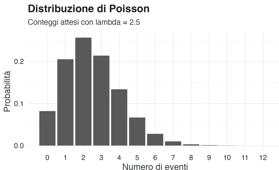
Figura 11.5: Funzione di massa di una distribuzione di Poisson con tasso medio pari a 2,5 eventi per intervallo.
