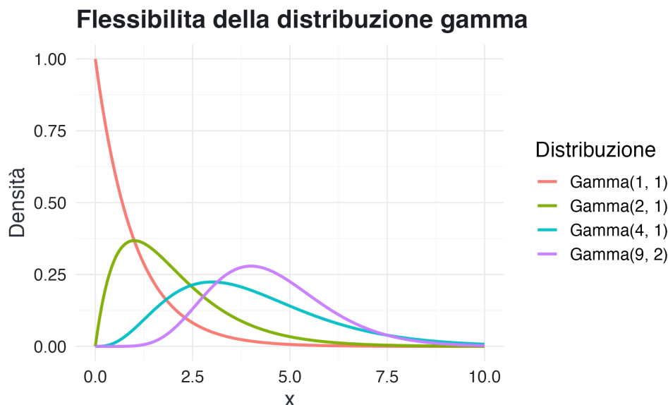
Figura 12.4: Esempi di distribuzioni gamma nella parametrizzazione shape-rate.
