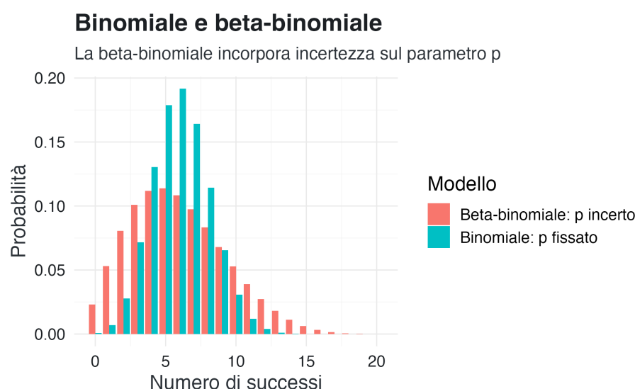
Figura 11.6: Confronto tra una binomiale con probabilità fissata a 0,30 e una beta-binomiale che integra una distribuzione di possibili valori di tale probabilità.
