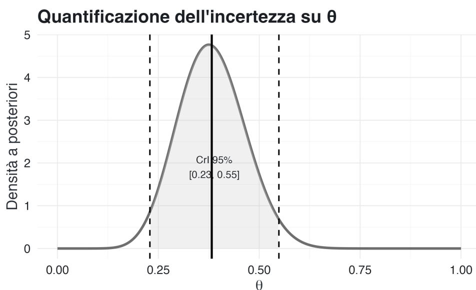
Figura 5.4: Distribuzione a posteriori con intervallo di credibilità al 95%.
