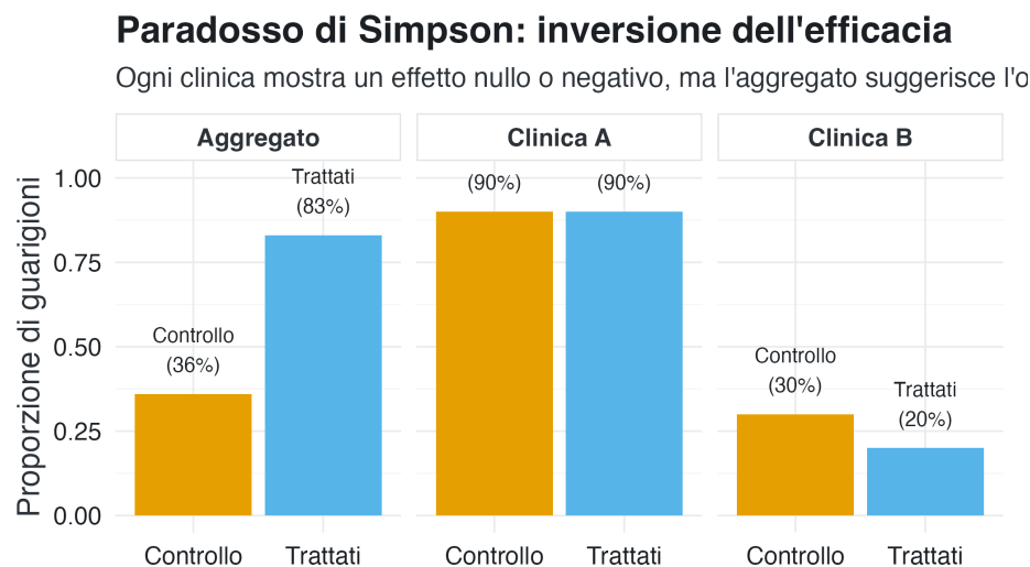
Figura 4.3: Un confronto aggregato può avere direzione diversa dai confronti effettuati entro ciascuna clinica.
