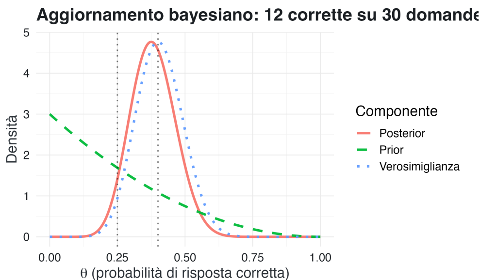
Figura 5.3: L'aggiornamento bayesiano nel modello Beta-Binomiale: il posterior è un compromesso tra prior e verosimiglianza.
