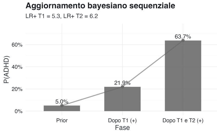
Figura 5.2: L'accumulo bayesiano di evidenze: ogni test positivo incrementa la probabilità.
