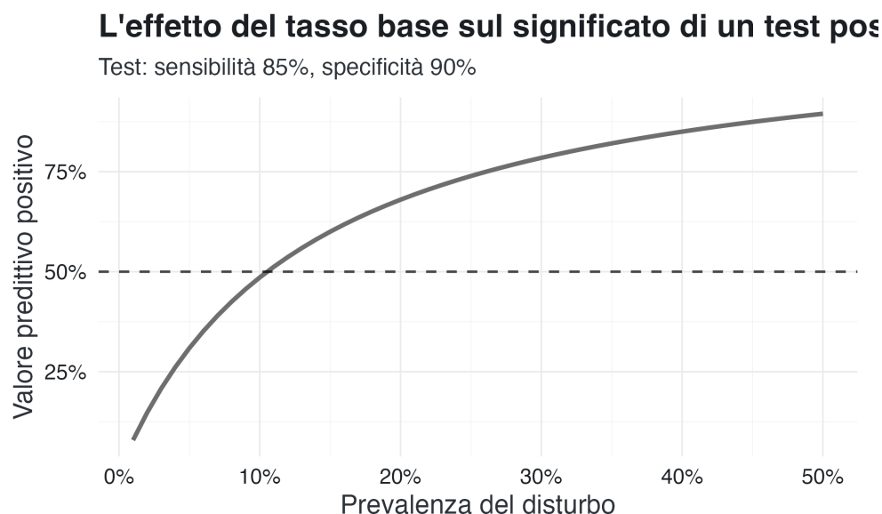
Figura 5.1: L'effetto della prevalenza sul valore predittivo positivo. Lo stesso test produce interpretazioni radicalmente diverse a seconda del contesto.
