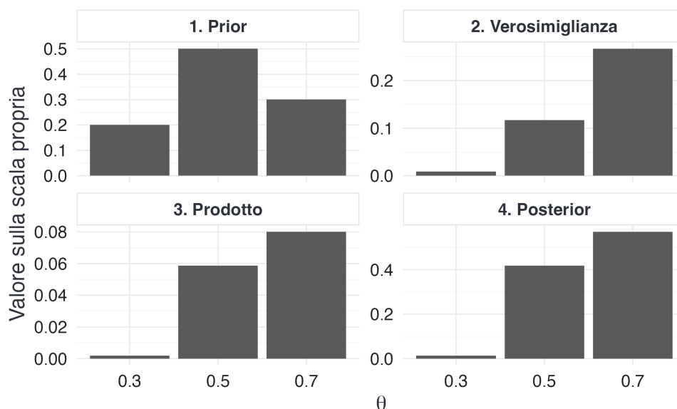
Figura 15.1: Aggiornamento bayesiano su tre valori possibili. Il prodotto punto per punto ripesa la prior; la normalizzazione produce la posterior. Le scale verticali sono separate perché le quattro quantità hanno ruoli differenti.
