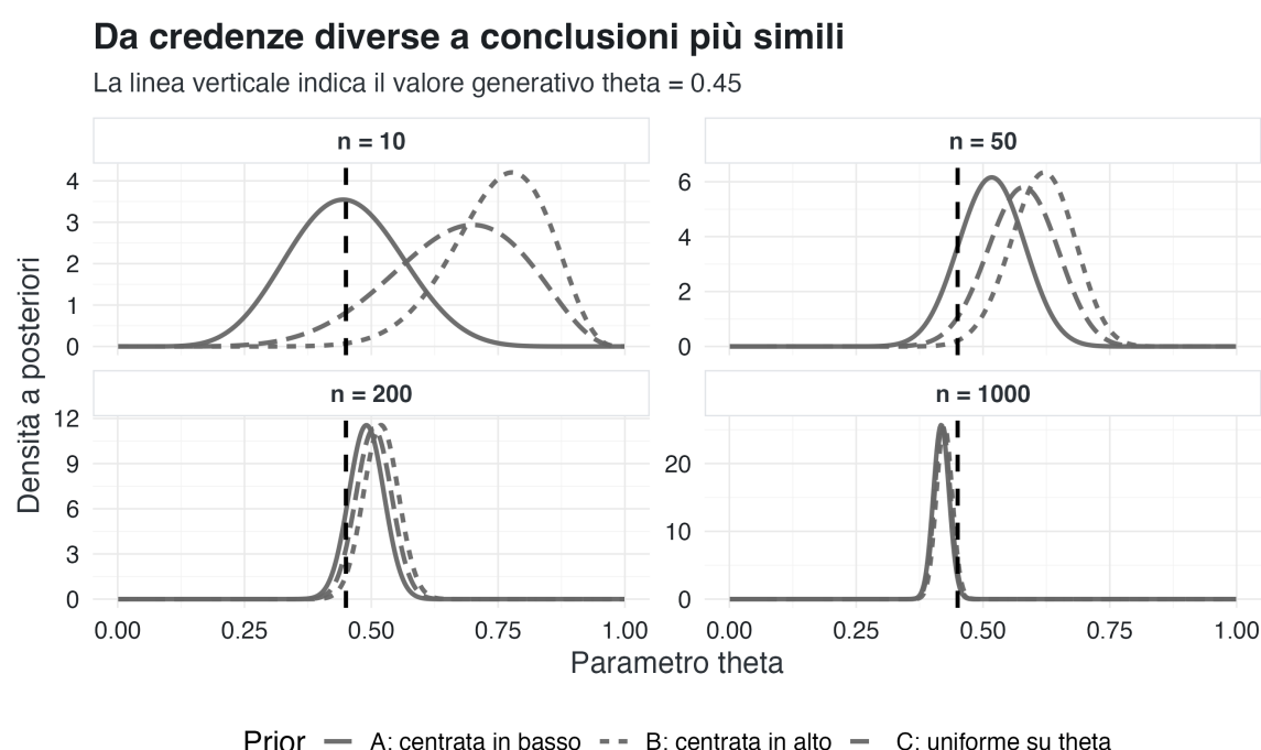
Figura 13.5: Distribuzioni posteriori ottenute con prior diverse ma con gli stessi dati cumulativi, al crescere della dimensione campionaria.
