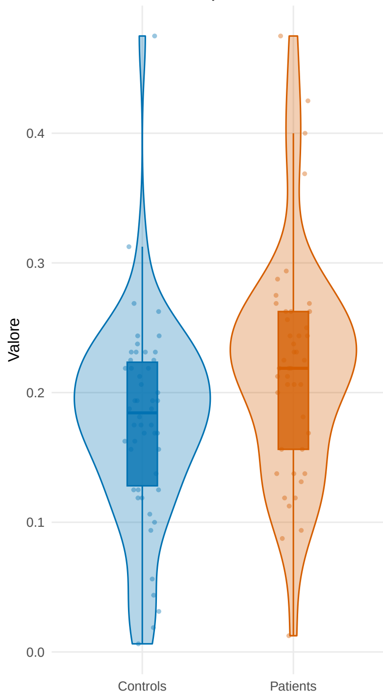
e_pers
