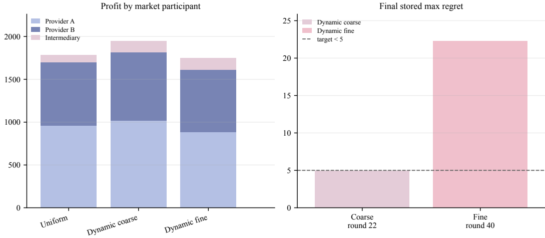
图 4: 利润组成与纯策略 regret 边界。左图按市场参与者（服务商 A、服务商 B 和中间商）分解利润，右图报告已保存候选的最佳响应 regret。粗网格快照达到 regret < 5，而细网格纯策略快照仍为 22.3，因此后者仅作为分辨率压力测试。
