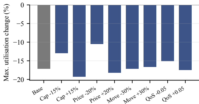
(b) Max. utilisation change (%)
