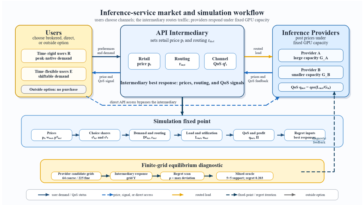
图 1: 市场结构。用户可以通过 API 中间商购买、直接连接服务商, 或退出市场。中间商依据价格和 QoS 在两个服务商之间路由流量。
