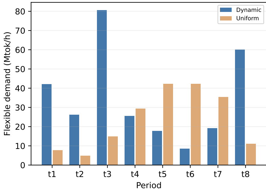
Flexible Demand Shift
