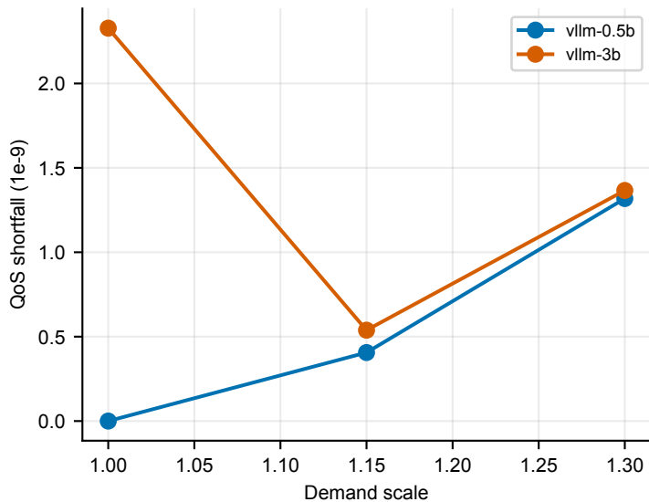
vLLM QoS substitution
