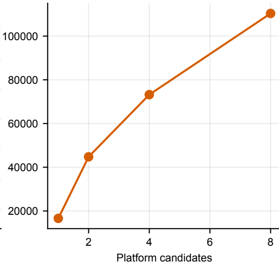
Function evaluations
