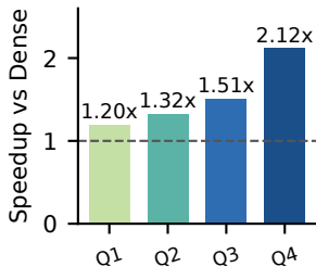
Copied-token quartile
