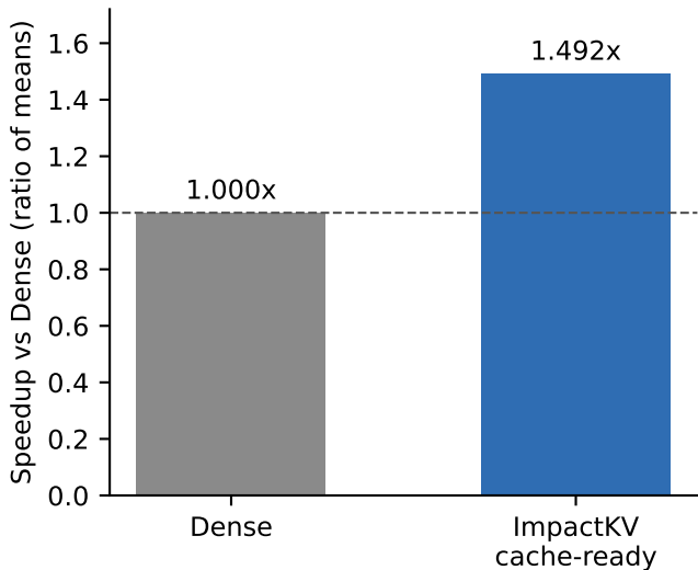
SWE-bench file-module TTFT (235 groups)
