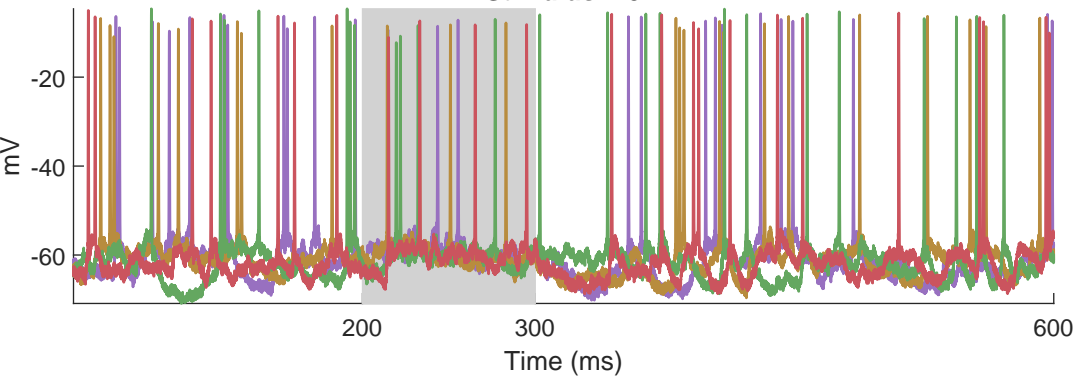
Stimulus: 13
