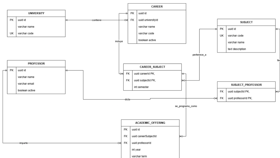
Figura 4: ApuntesUCT - MER Catalog Service.
