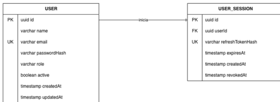
Figura 3: ApuntesUCT - MER Auth Service.
