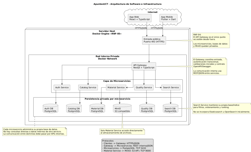
Figura 1: ApuntesUCT - Diagrama de Arquitectura de Software.
