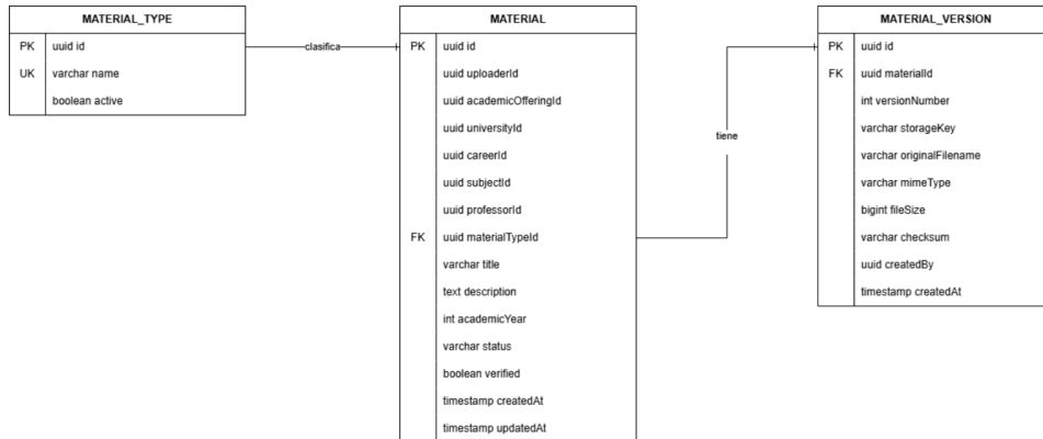
Figura 5: ApuntesUCT - MER Material Service.
