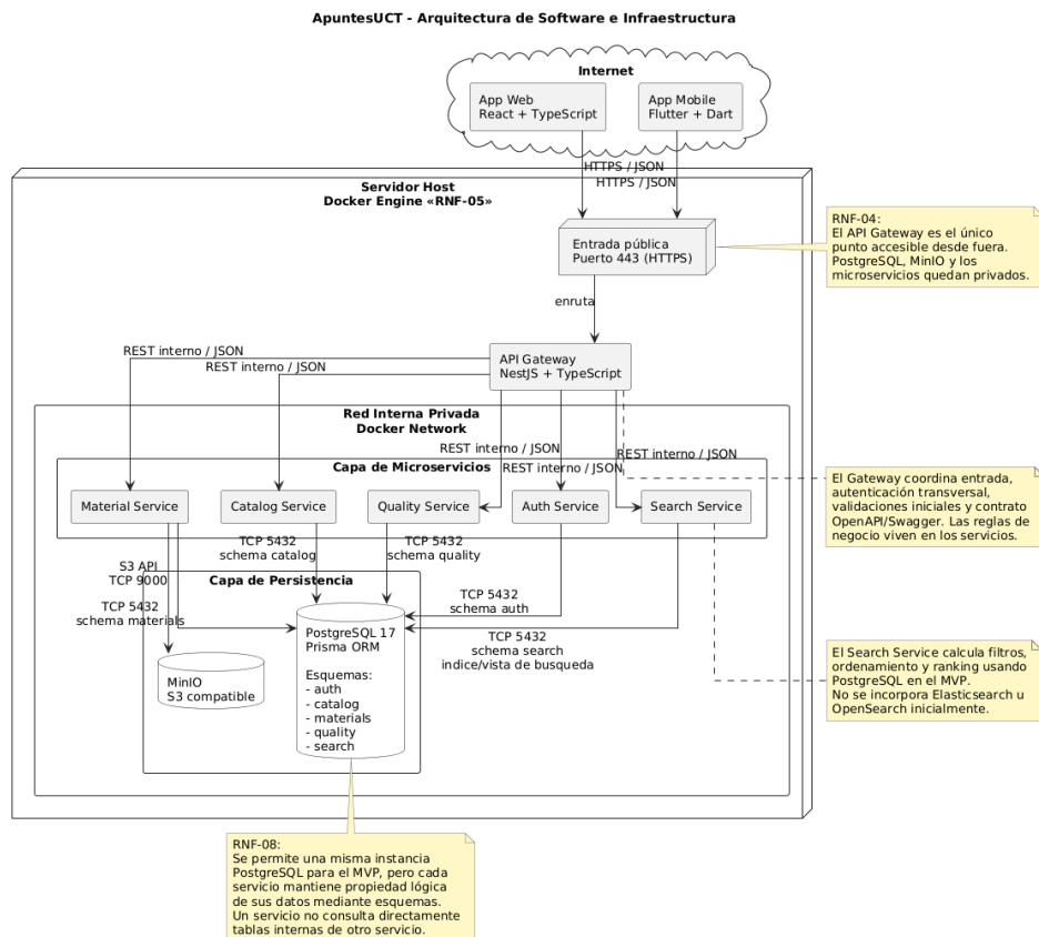
Figura 1: ApuntesUCT - Diagrama de Arquitectura de Software.
