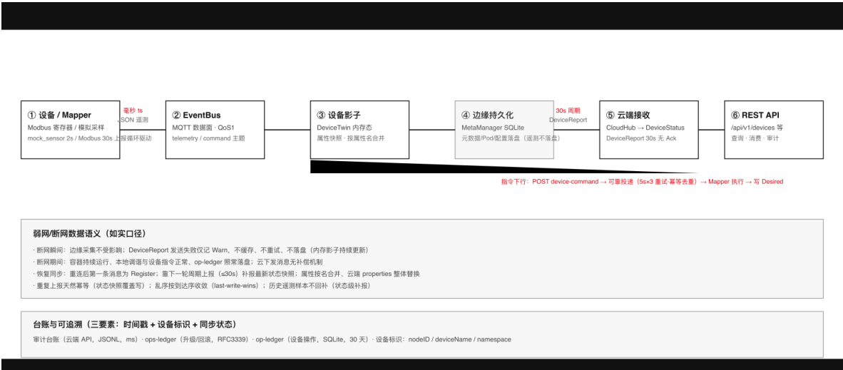
图 6.1: EdgeFlow 数据全链路
