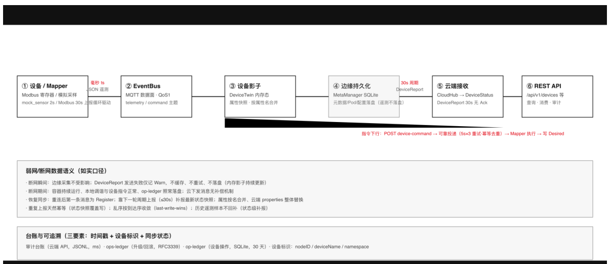
图 6.1: EdgeFlow 数据全链路
