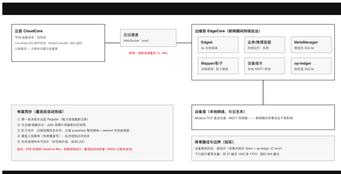
图 3.1: 弱网自治场景部署拓扑
