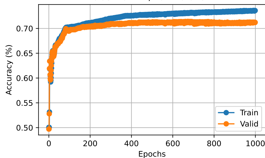
Epochs= 1000, N_{layers} = 3 bias= 0.100, var= 0.0272
