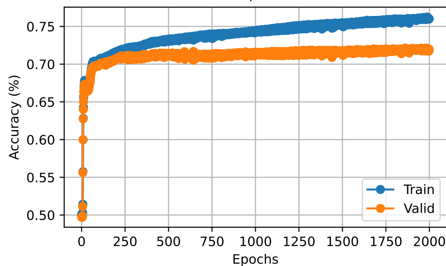
Epochs= 2000, N_{layers} = 4 bias= 0.079, var= 0.0432
