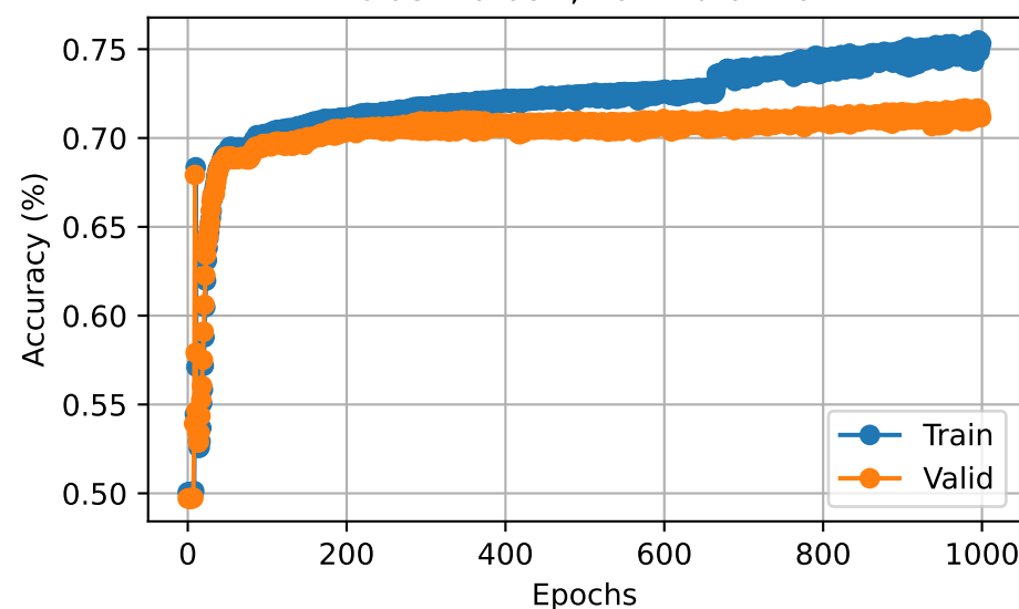
Epochs= 1000, N_{layers} = 5 bias= 0.097, var= 0.0416
