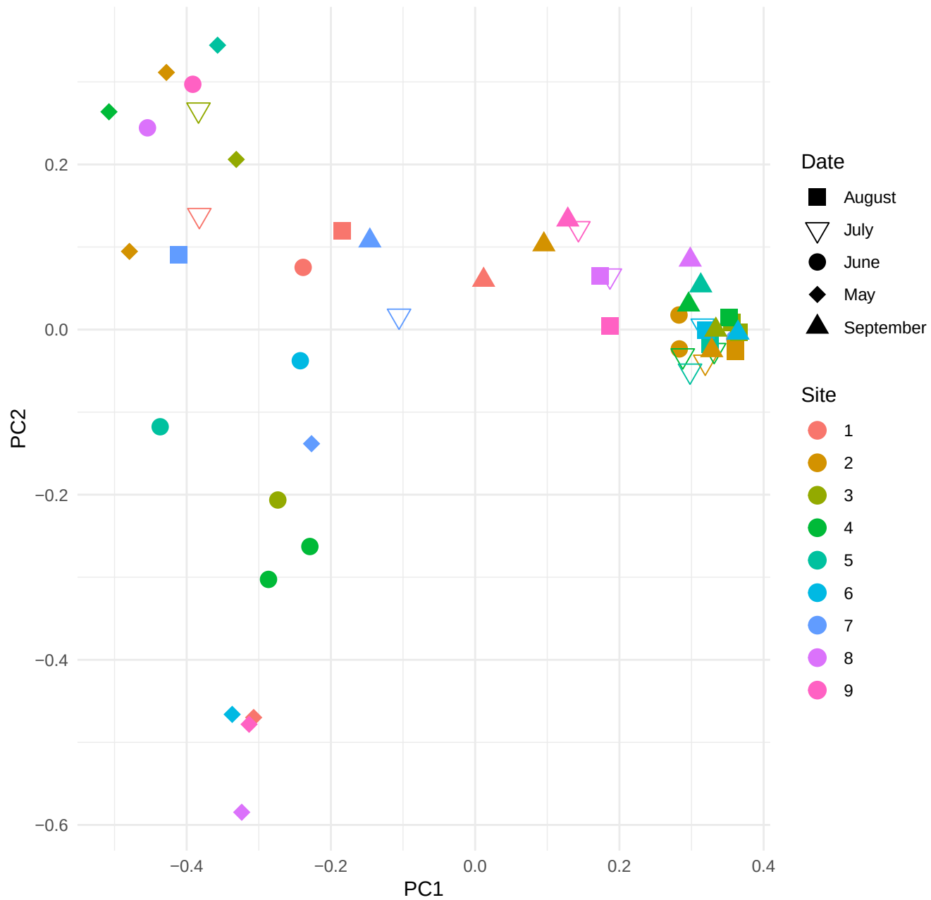
16s Bray Curtis PCA
