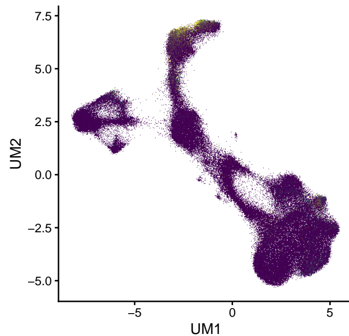
FPR1 (0–3.8)
