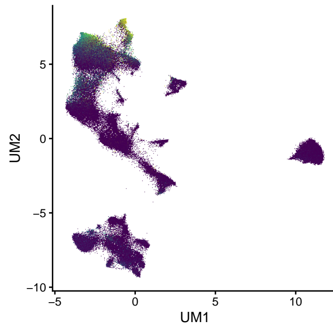
ANXA4 (0–4.9)
