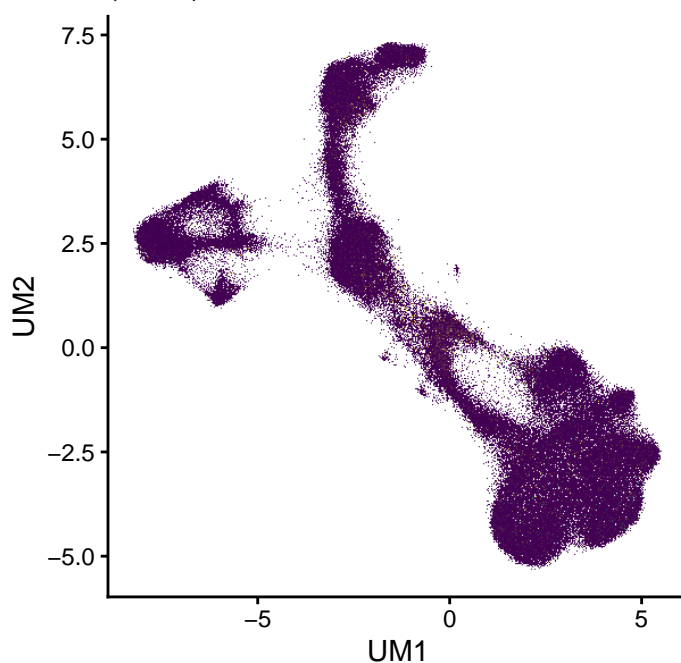
NKG7 (0–4.7)
