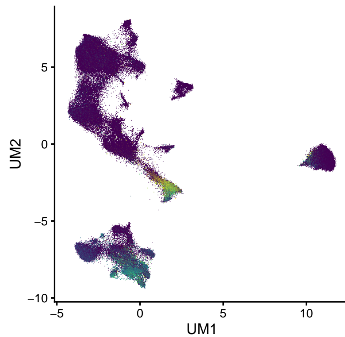
ANXA4 (0–4.9)
