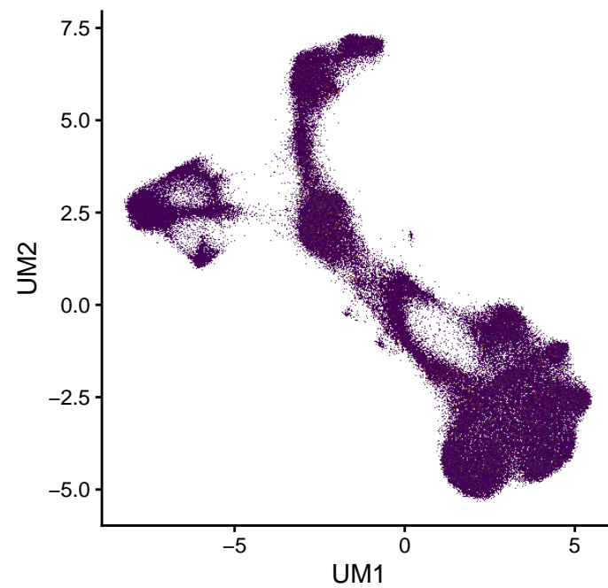
FPR1 (0–3.8)
