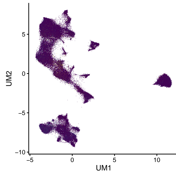
NKG7 (0–3.9)
