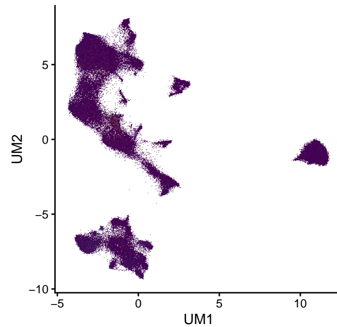
NKG7 (0–3.9)
