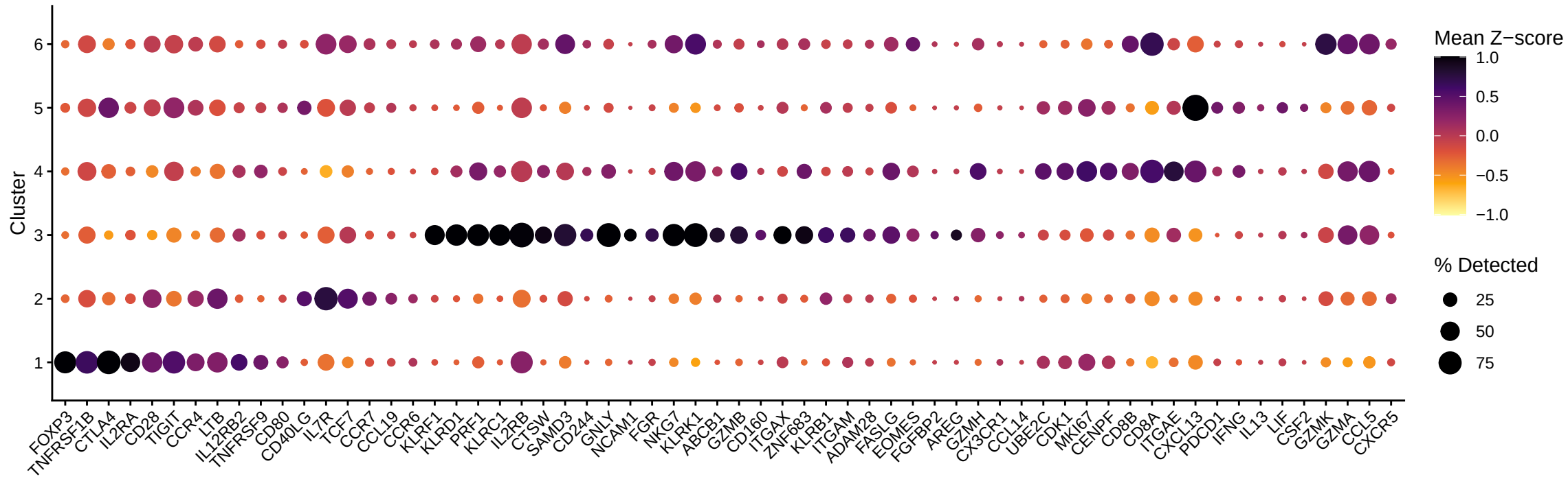
DE Markers
