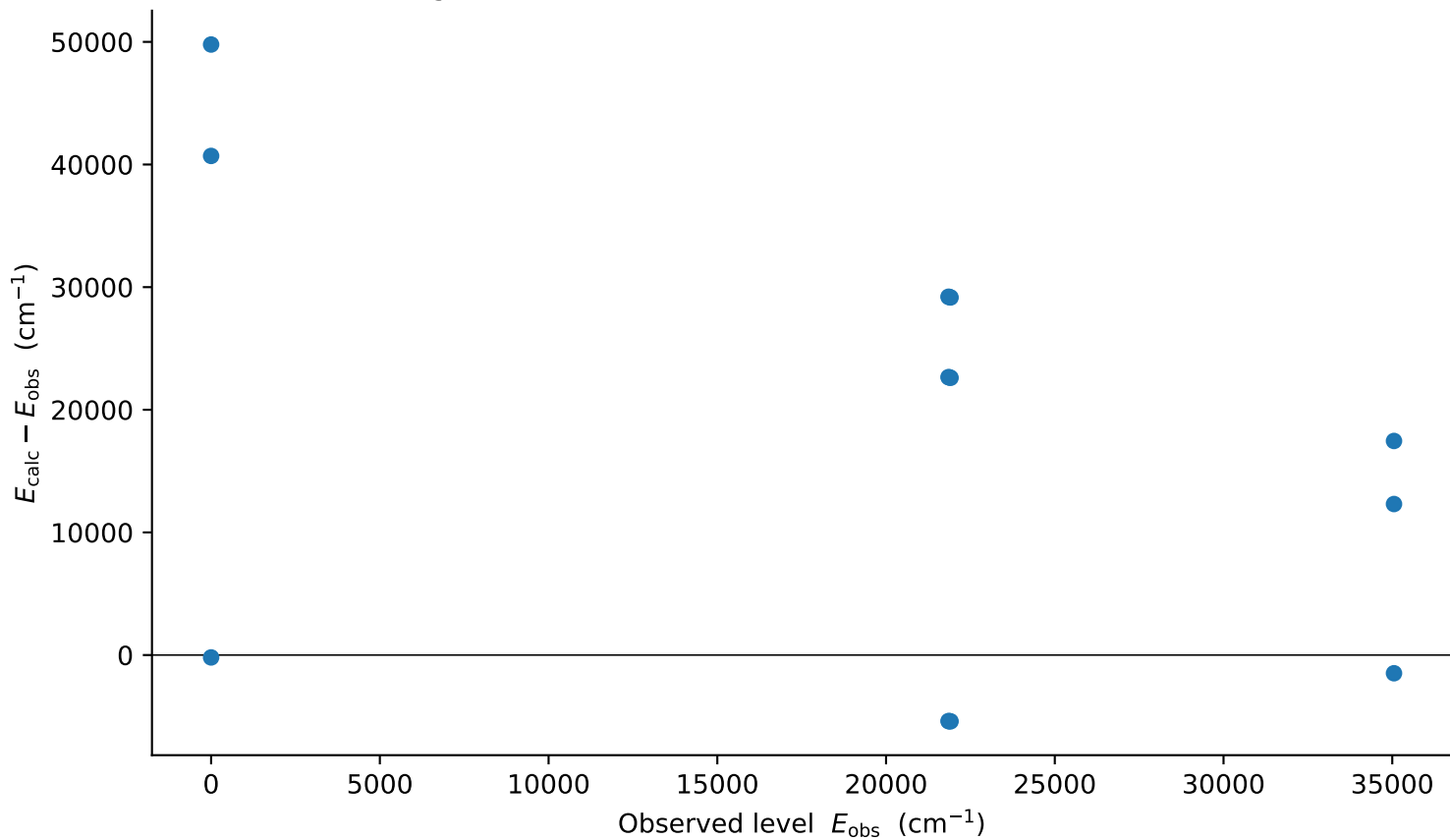
Mg I: level-fit residuals (RMS = 24186 cm -1 , ab initio)
