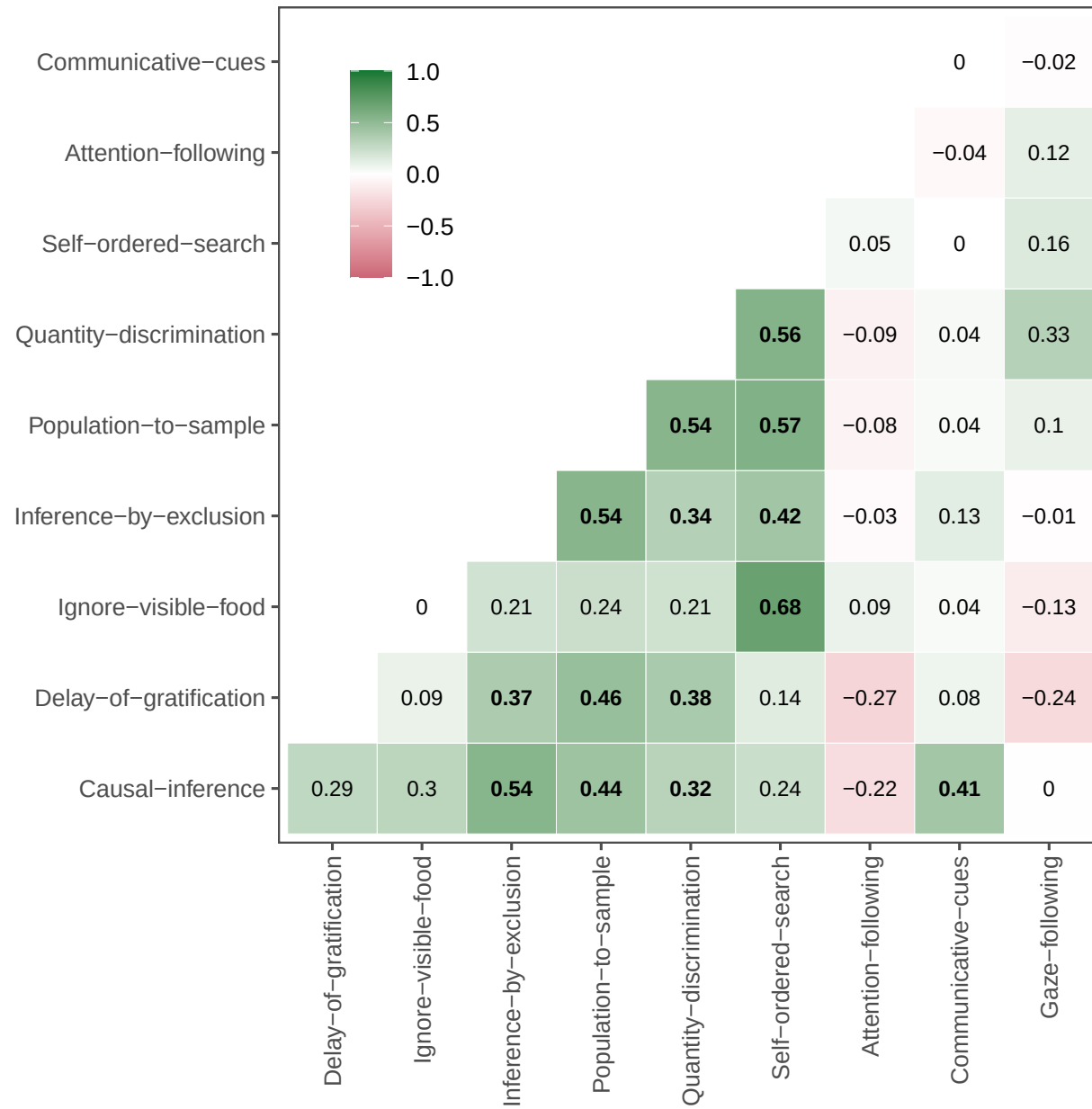
Pairwise brms binomial model
