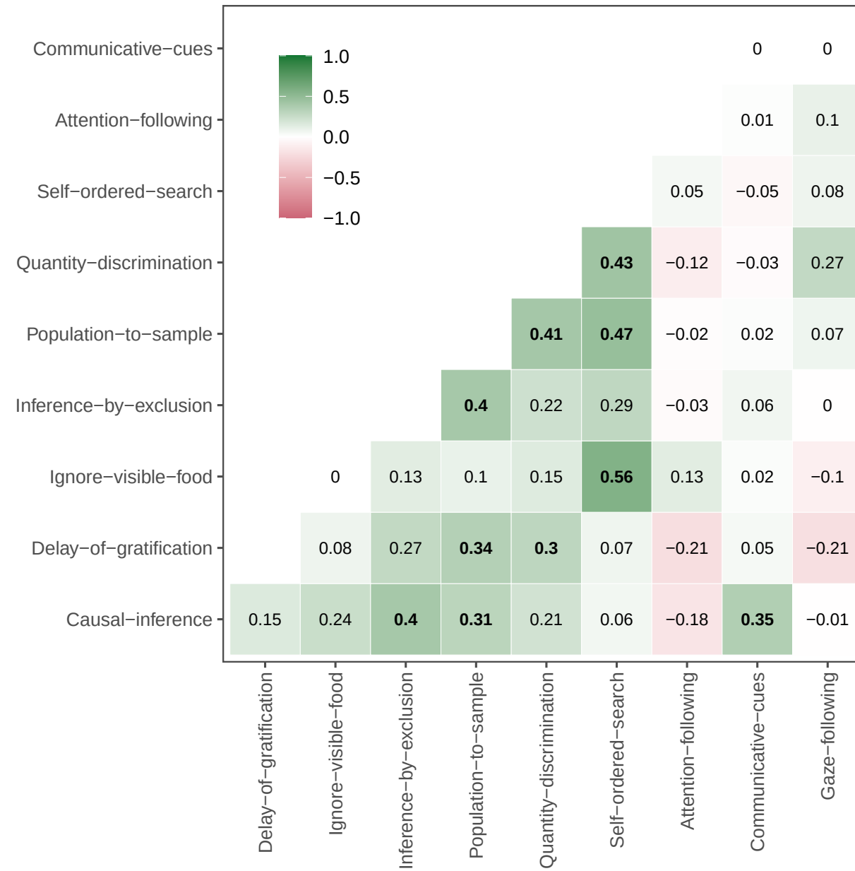
brms binomial model
