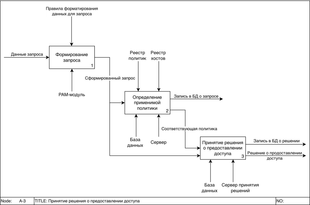
Рисунок 8 – Модель дочерней работы «Принятие решение о предоставлении доступа»
