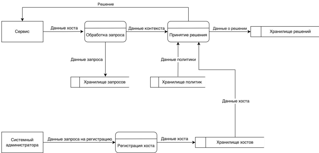
Рисунок 4 – Логический уровень DFD диаграммы
