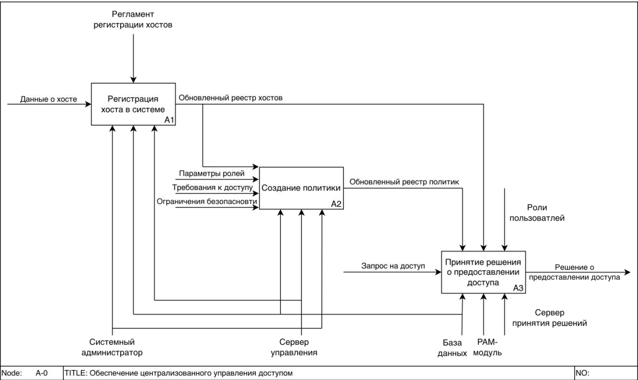
Рисунок 7 – Диаграмма декомпозиции
