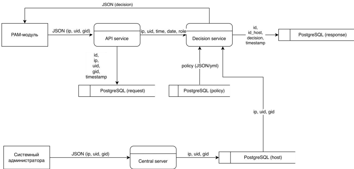
Рисунок 5 – Физический уровень DFD диаграммы
