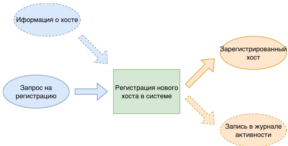
Рисунок 2 – Схема окружения бизнес-процесса по регистрации нового хоста в системе
